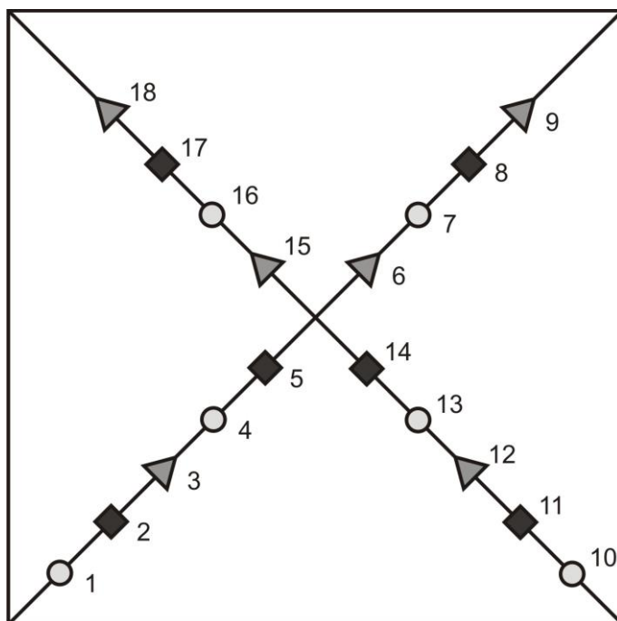
Рисунок А.1 – Схема отбора проб почвы (грунта)
